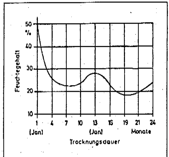
Diagramm Wassergehalt
