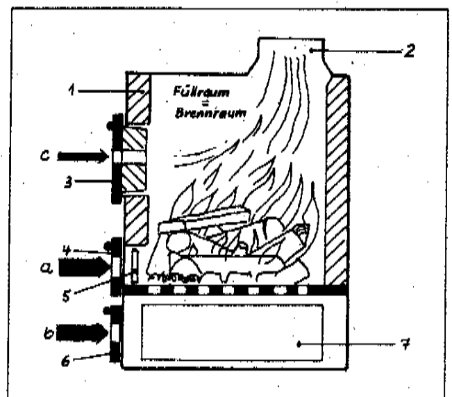
Bild 1: Ofen bzw. Kachelofeneinsatz mit oberem Abbrand
